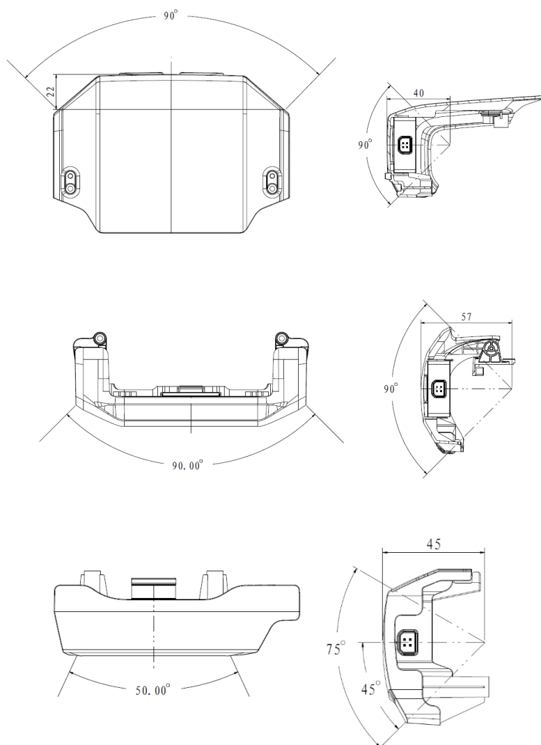
图 3-10 装甲安装规范示意图
