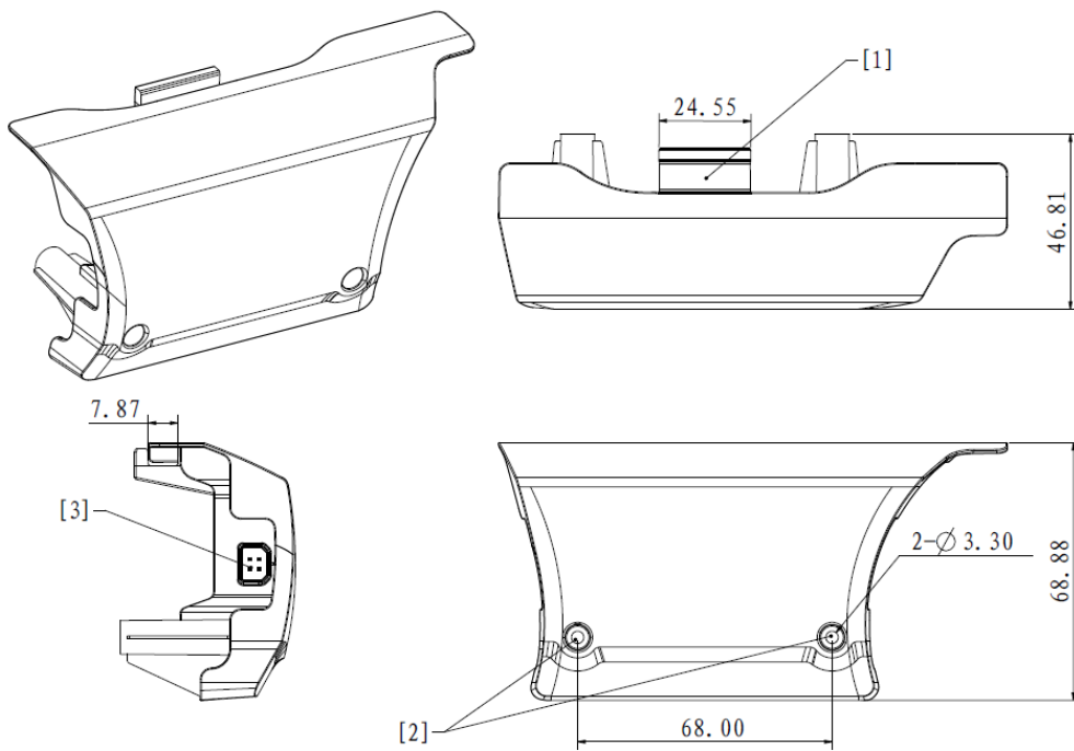
图 3-5 右装甲模块示意图
