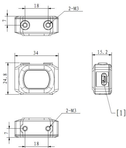
[1] 运动控制器 CAN BUS 接口
