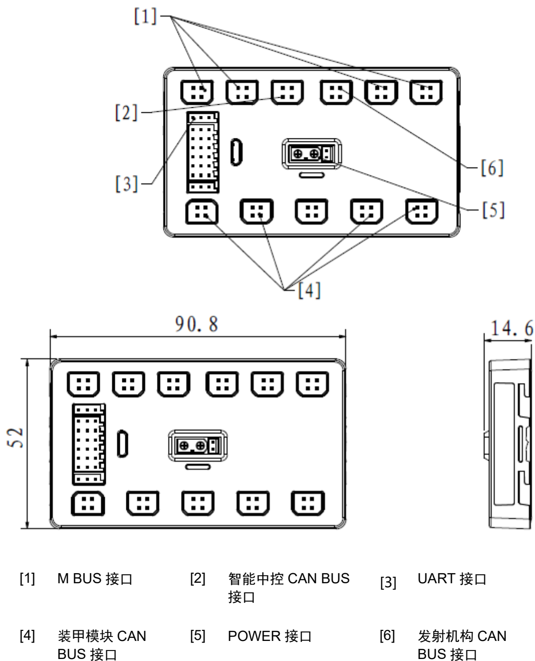
图 3-1 运动控制器模块
